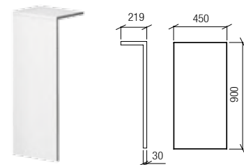
01 Vorsatzblende aus weiß beschichtetem Holzwerkstoff, mit umlaufendem Profil, aus schwarz pulverbeschichtetem Stahl
